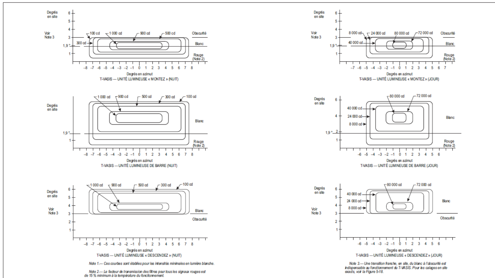
Figure A2-22. Répartition de l'intensité lumineuse du T-VASIS et de l'AT-VASIS
