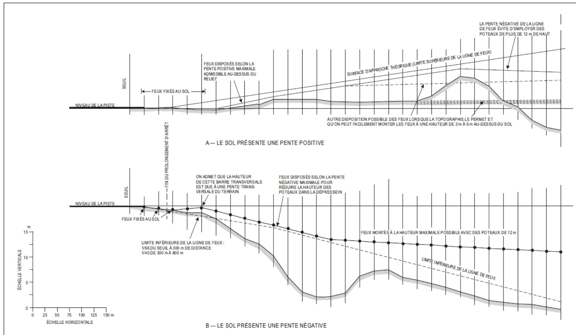
Figure A-9. Tolérance verticale d'installation
