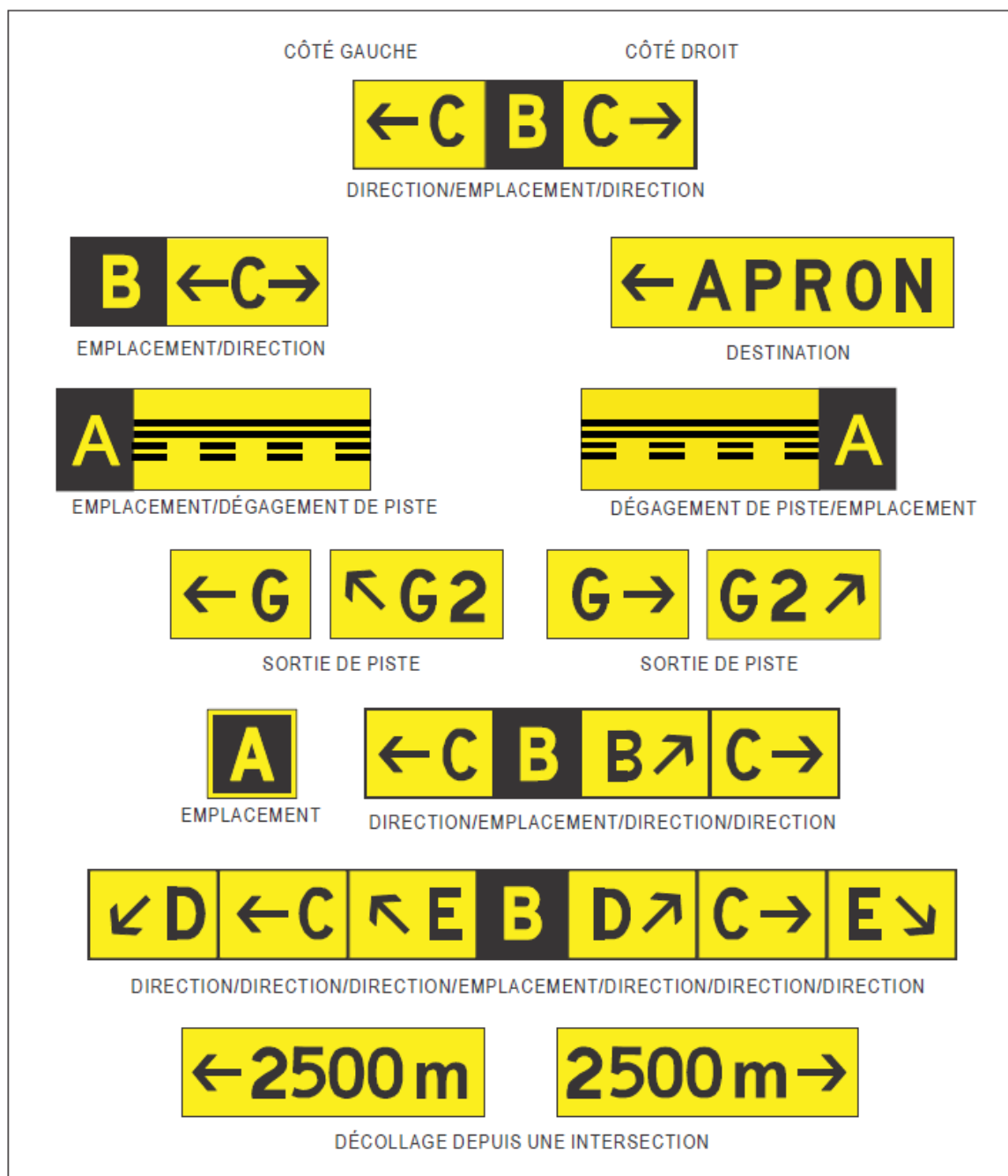
Figure 5-31. Panneaux d'indication
