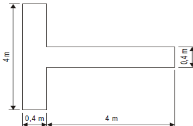
Figure 5-1. Indicateur de direction d'atterrissage
