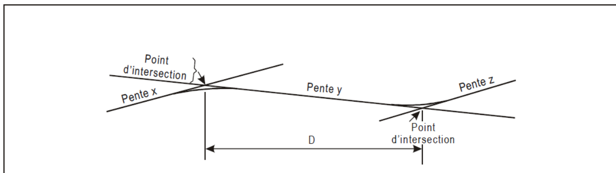
Figure A-2. Profil de l'axe de piste
