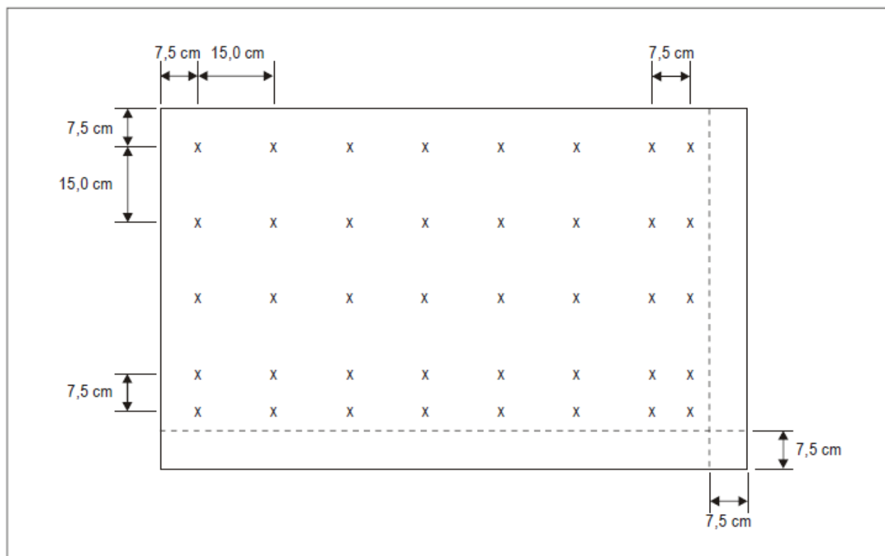
Figure A4-1. Points de grille pour calculer la luminance moyenne d'un panneau de signalisation
