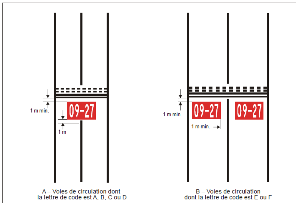
Figure 5-10. Marque d'obligation
