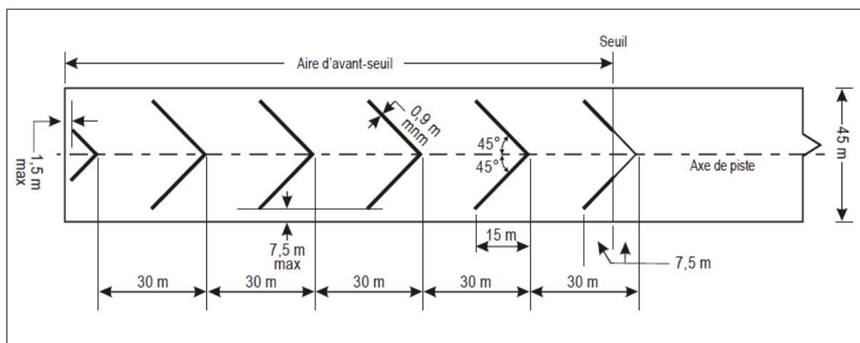
Figure 7-2. Marques d'avant-seuil
