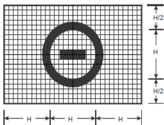
Panneau D'ENTRÉE INTERDITE
