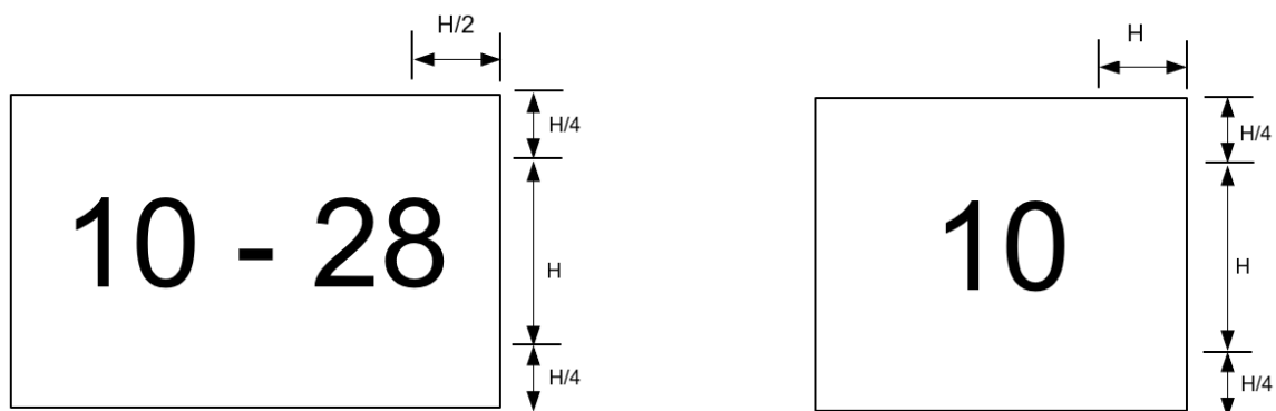
A. Panneau à deux indicatifs de piste
