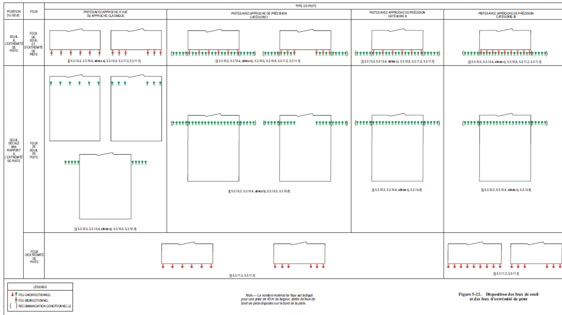
Figure 5-22. Disposition des feux de seuil et des feux d'extrémité de piste
