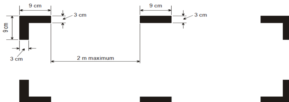
INDICATION DES ZONES DE PÉNÉTRATION DU FUSELAGE (voir § 2.4.2.6)
